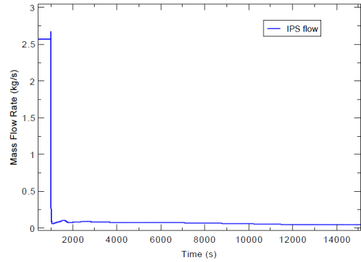
شکل ۸: آهنگ عبور جریان خنک کننده از IPS در سناریو ۳ حادثه LOFA
