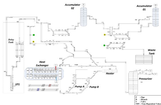
شکل ۱: گره بندی تست لوپ راکتور تهران برای مدل سازی در کد RELAP5
