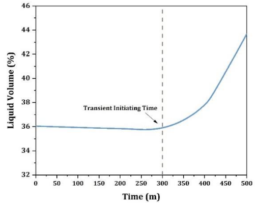
شکل ۵: تغییرات درصد حجم مایع درون سیستم تعدیل فشار
