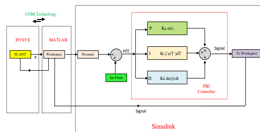
شکل ۳: نمایی از فرآیند کنترل کننده PID در سیمولینک متلب
